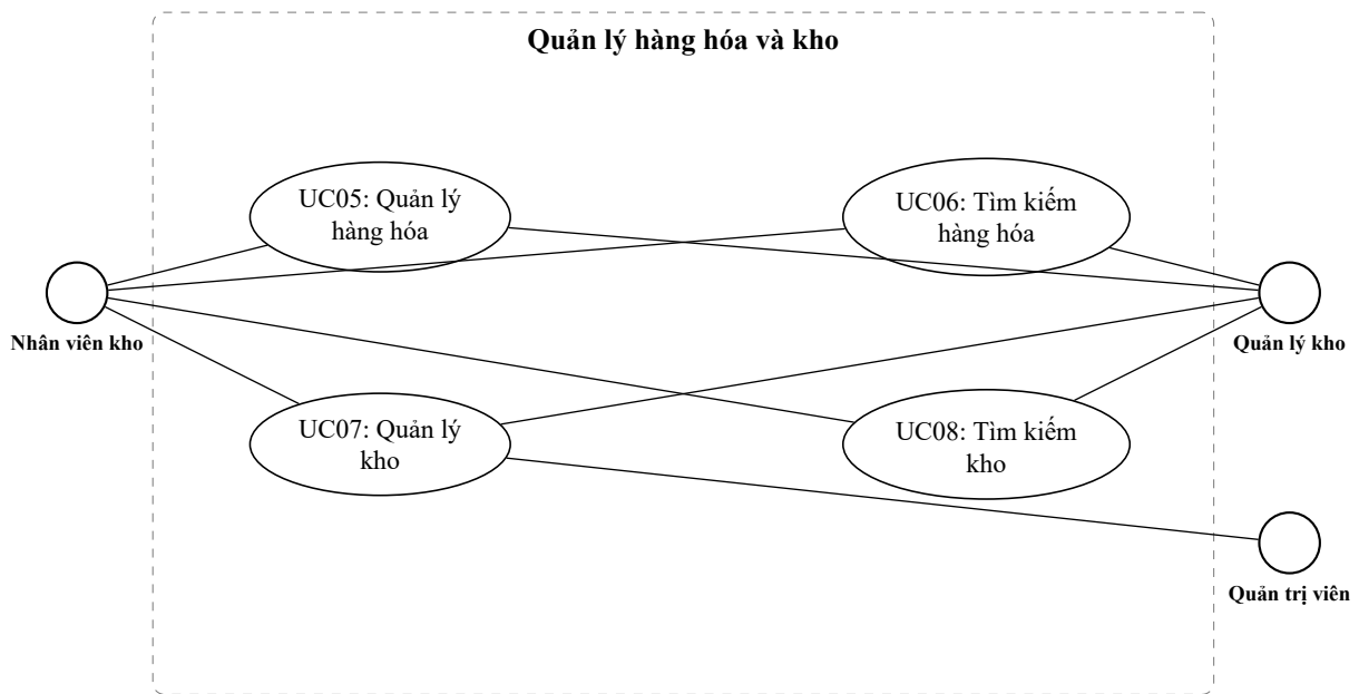
Hình 1: Sơ đồ use case phân rã – Quản lý hàng hóa và kho
